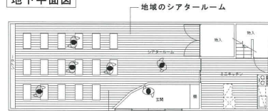
地下平面図
